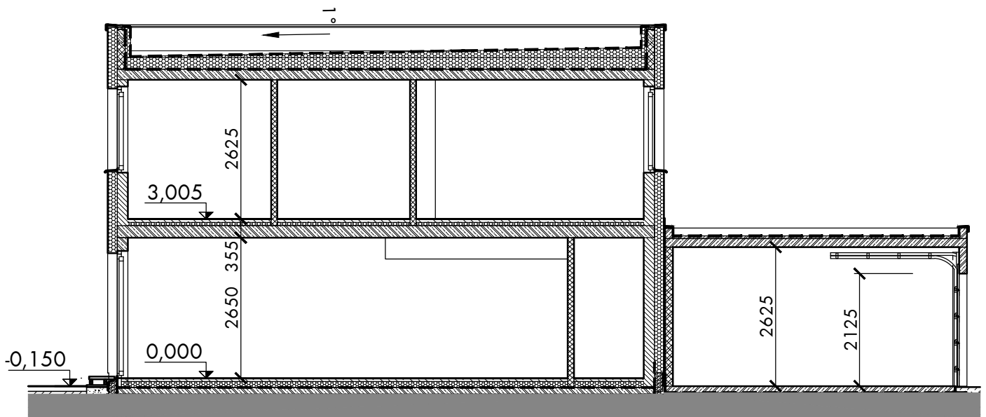
ŘEZ PODÉLNÝ
